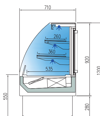
VSAD-6-9-C VSAD-6-13-C
